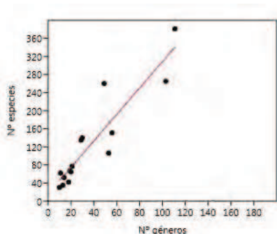
Fig. nº 1. Gráfica de la relación entre el número de géneros y número de especies y su correspondiente recta de regresión lineal, para los datos de las 15 familias de la flora vascular valenciana que poseen más de 10 géneros.
